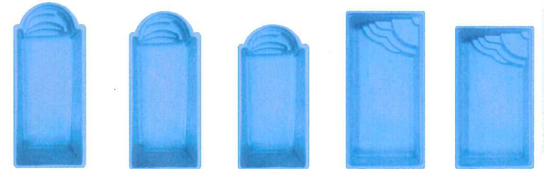
BARBADE* Hors tout : 10.10 m x 4.00 m Profondeur : 1.53 m SAMOA* Hors tout : 9.30 m x 4.00 m Profondeur : 1.53 m TEVA* Hors tout : 7.50 m x 4.00 m Profondeur : 1.53 m TRINITÉ** Hors tout : 10.20 m x 4.20 m Profondeur : 1.50 m FLORES** Hors tout : 8.20 m x 4.20 m Profondeur : 1.50 m
