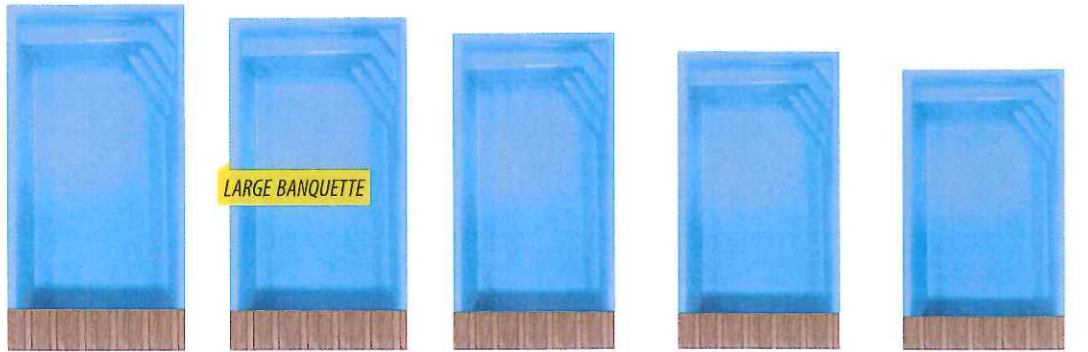
COMORES** Hors tout : 10.20 m x 4.20 m Profondeur : 1.50 m CALYPSO** Nouveauté! LARGE BANQUETTE Hors tout : 9.20 m x 4.20 m Profondeur : 1.50 m CAP HORN** Hors tout : 8.15 m x 3.55 m Profondeur : 1.50 m AMBRE* Hors tout : 7.30 m x 3.55 m Profondeur : 1.50 m MAHE* Hors tout : 6.30 m x 3.55 m Profondeur : 1.50 m
